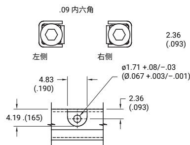
安装孔细节展示 不按比例
