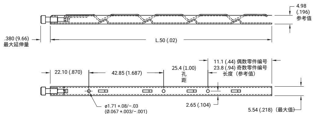
安装孔细节展示 不按比例
