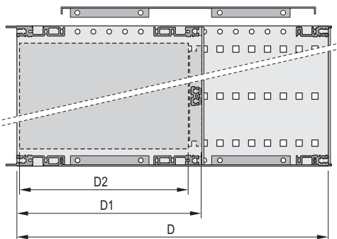
D = Gesamttiefe, D1=Stecktiefe, D2=Leiterplattentiefe = D1 - 15 mm
