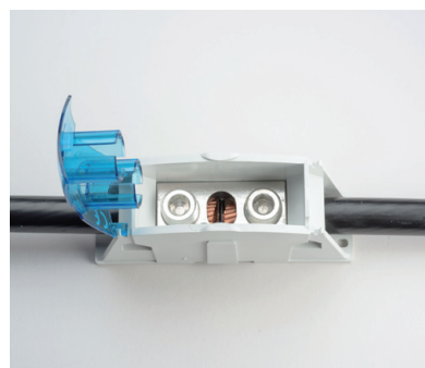
Système breveté de maintien des vis de fixation
