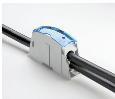
Raccordement par deux Câbles
