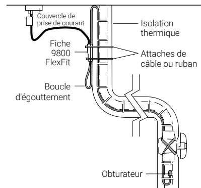
Figure 1. Installation type d'habitation préfabriquée
