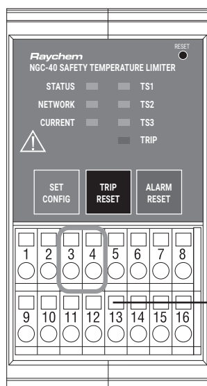
Rys. 6: Zaciski alarmowe
