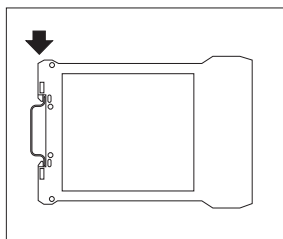
Rys. 2: Montaż modułu NGC-40-SLIM na szynie DIN
