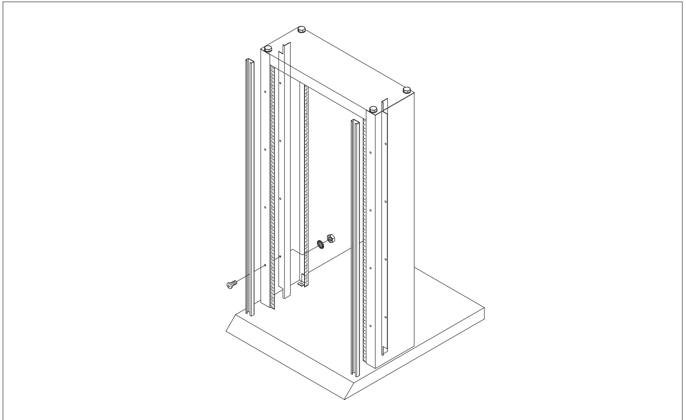
Montageprofil 19"-Rasterprofil
