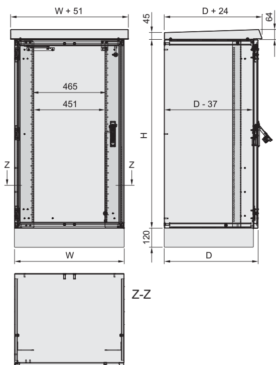
Version avec socle hauteur d'ouverture de porte = H - 75 mm; largeur d'ouverture de porte = W - 75 mm
