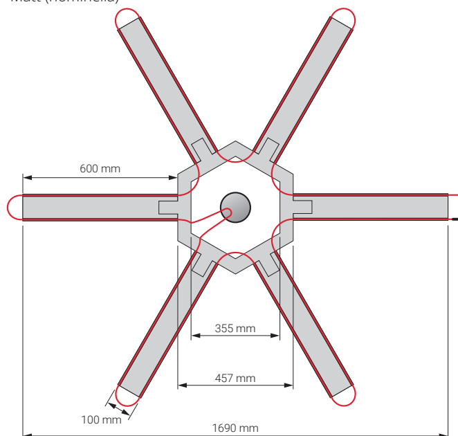
Mått (nominella)
