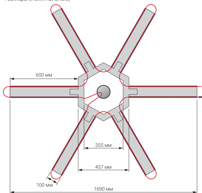
Размеры (номинальные)
