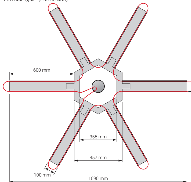
Afmetingen (nominaal)
