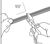
Kapa värmekabeln i rak vinkel
