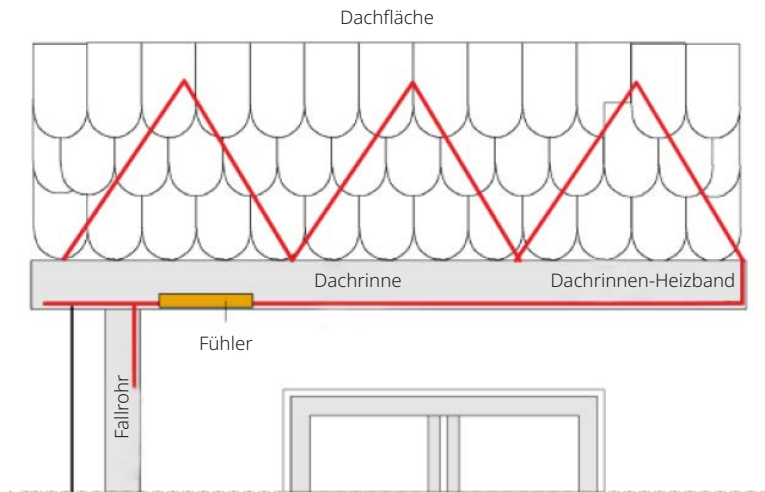
Einbau des Fühlers (Seitenansicht).
