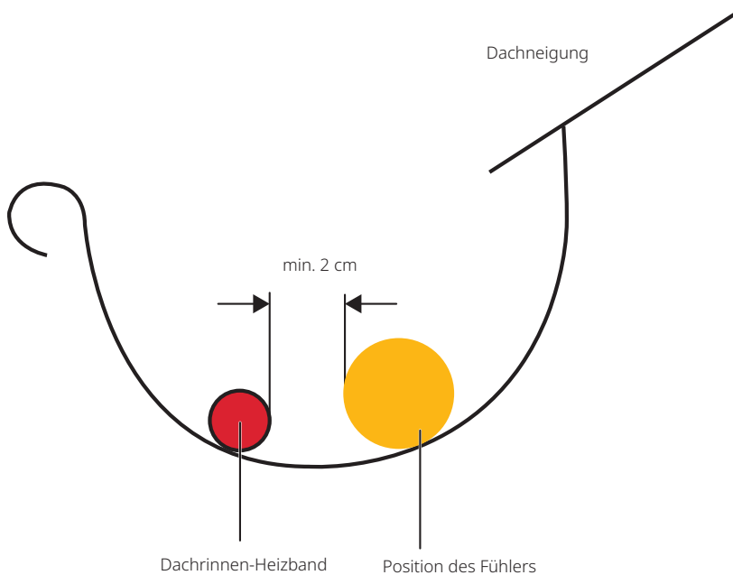
Installation des Fühlers (Ansicht der Dachrinne).
