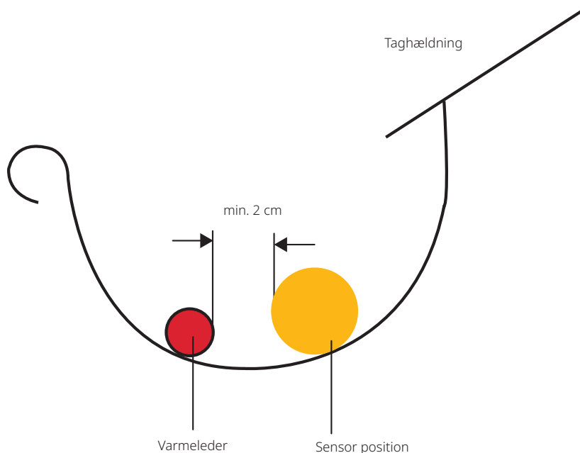
Installation af sensor (set fra siden).
