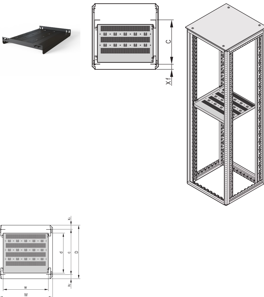
Ripiano Varistar 19", fisso, 75 kg.
