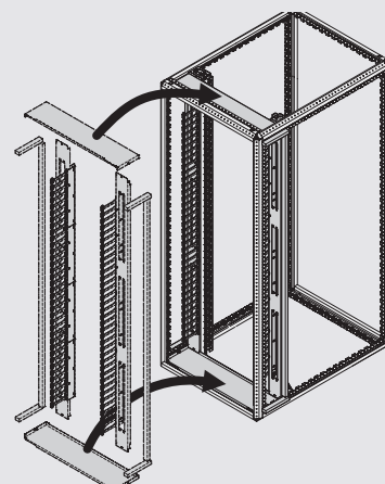
Bandeaux standard avec découpes et peignes guide-câbles
