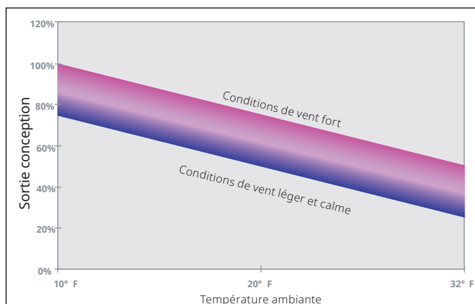
Performances du système HECS pour différentes températures ambiantes et conditions de vent
