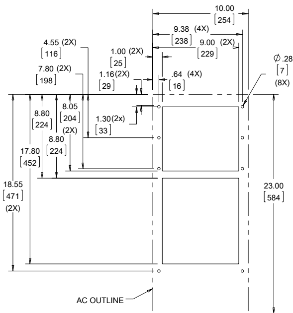
Cutout Dimensions
