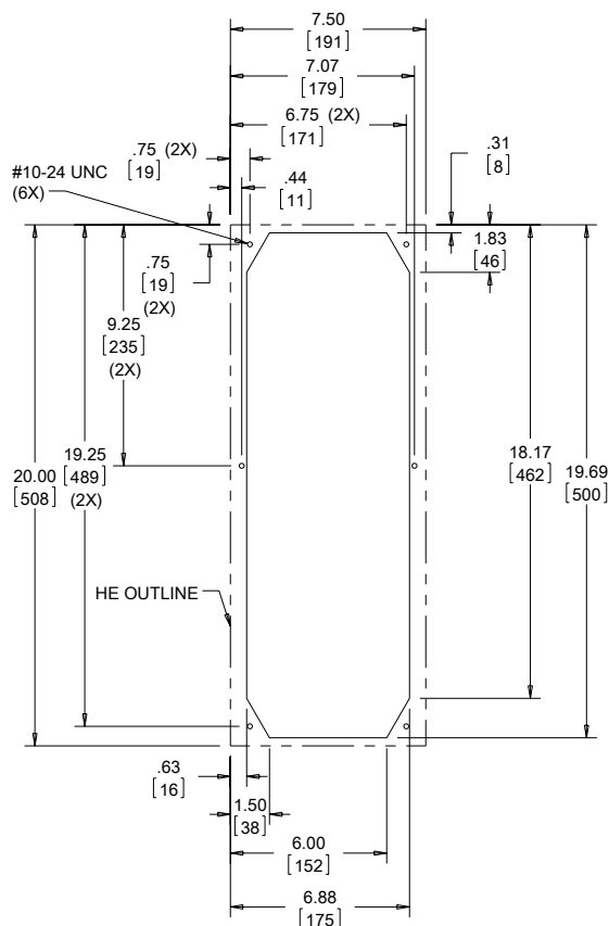
Cutout Dimensions
