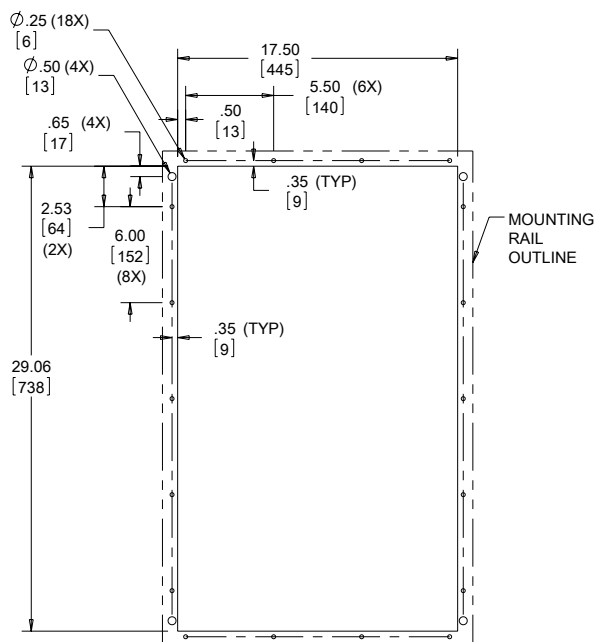
Cutout Dimensions
