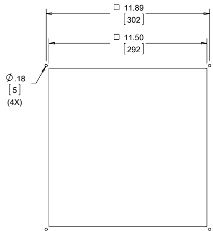
Cutout Dimensions
