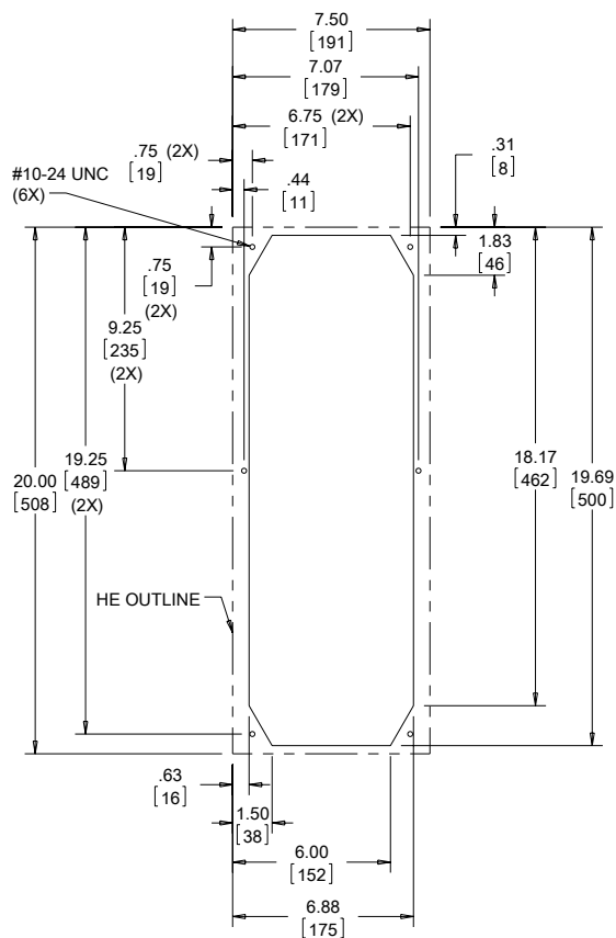
Cutout Dimensions
