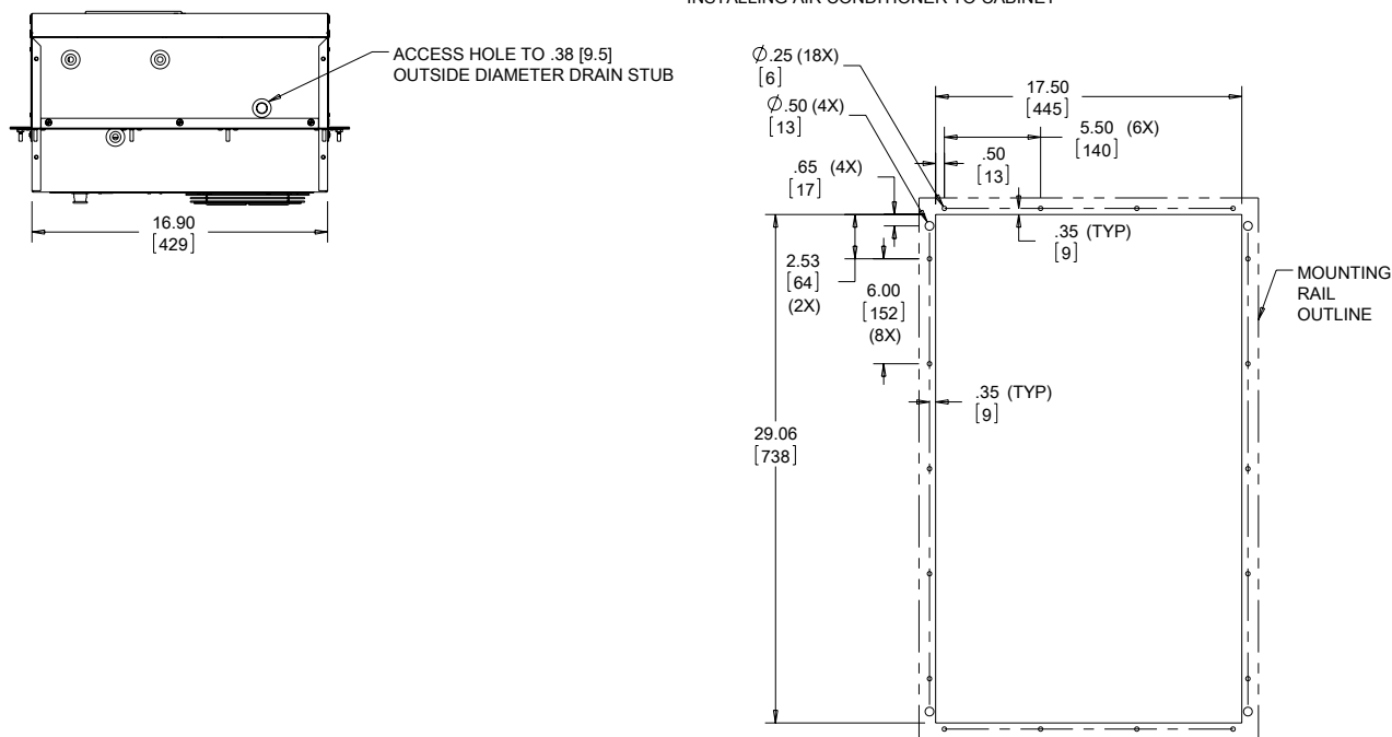
Cutout Dimensions
