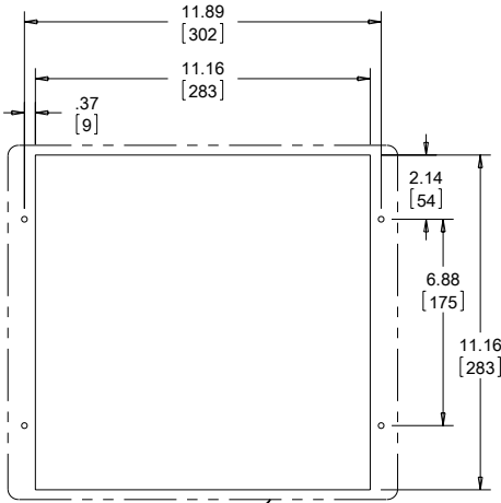
CUTOUT DIMENSIONS
