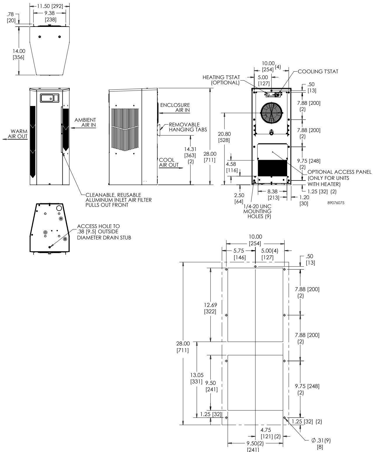
Cutout Dimensions
