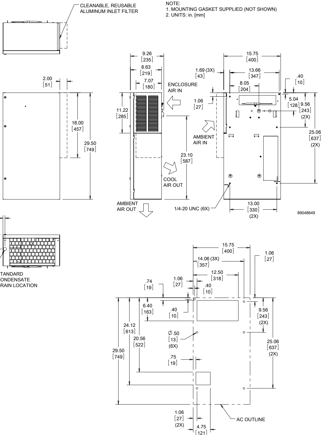
Cutout Dimensions
